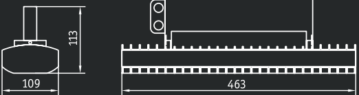
Габарит корпуса 228 (225 Вт)
