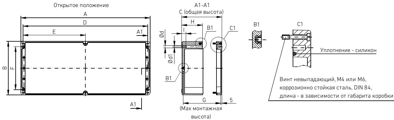
Габаритные и установочные размеры
