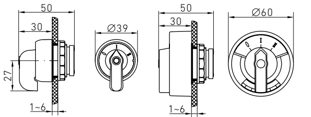
Компактная ручка типа SH Ручка переключателя типа LH
