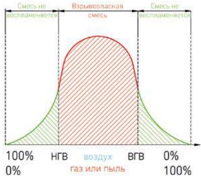
График 1. Области формирования взрывоопасной смеси
