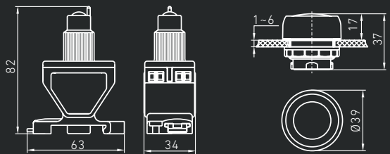
Габаритные размеры взрывозащищенного индикаторного блока
