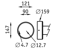
Установочные размеры
