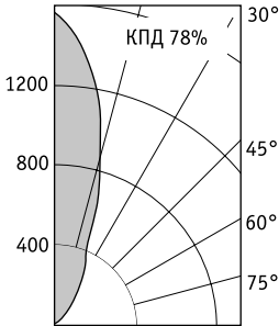
NFG 40 P75
