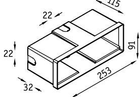
Монтажный бокс
