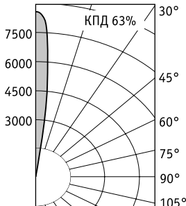
NFG 51 HG70 (12°)
