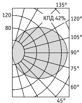
NBR 41 F118
