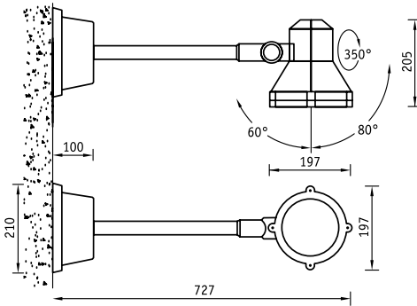
NBS 20 HG70 12°
