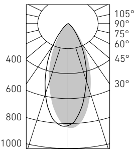
WASHLINE MINI LED 12 (40)
