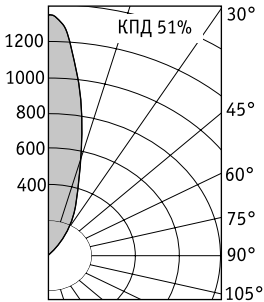
NFG 60 HG70 (26°)
