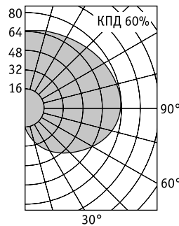
NBL 52 H70
