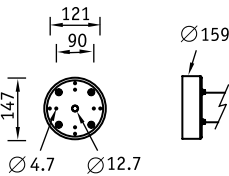
Установочные размеры
