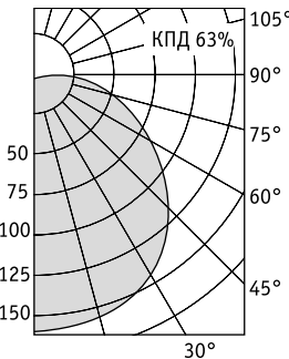
STAR NBT 11 F126
