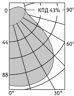
NBL 11 H70
