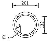
NBS 21 HG70 26°
