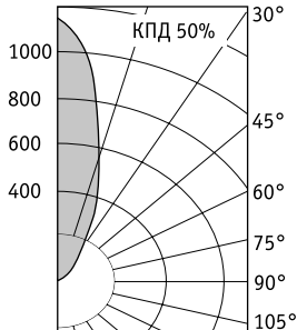
NFG 51 HG70 (26°)
